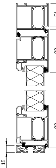
DoorPro 70RC, Profile Dimensions
